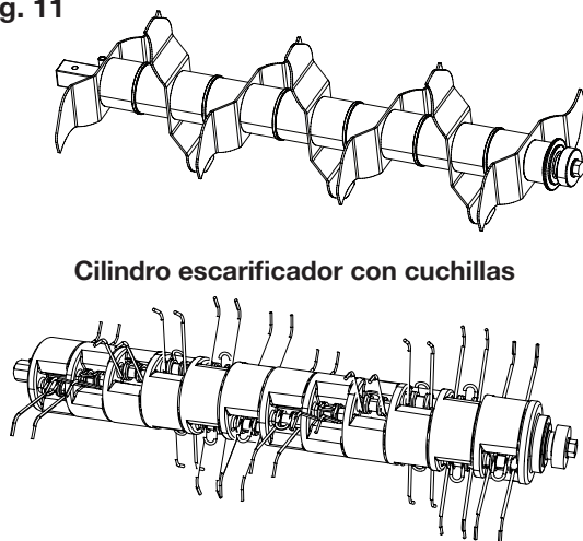
Cilindro rastrillador (aireador) con púas metálicas flexibles
