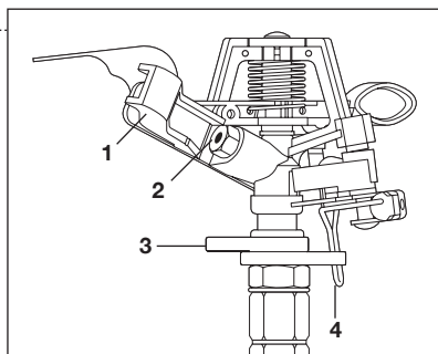
Tête d'arrosage
