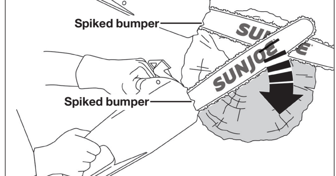
Fig. 19D
